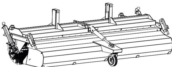
Configuratie 3: Bema 20 Dual Vuilopvangbak Dual hydraulisch, incl. 3e steunwiel Spindelborstel verstelling Mogelijkheid om te vegen met bak open
