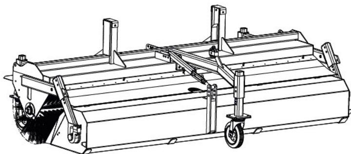
Configuratie 1: Bema 20 vuilopvangbak mechanisch + 3e steunwiel
