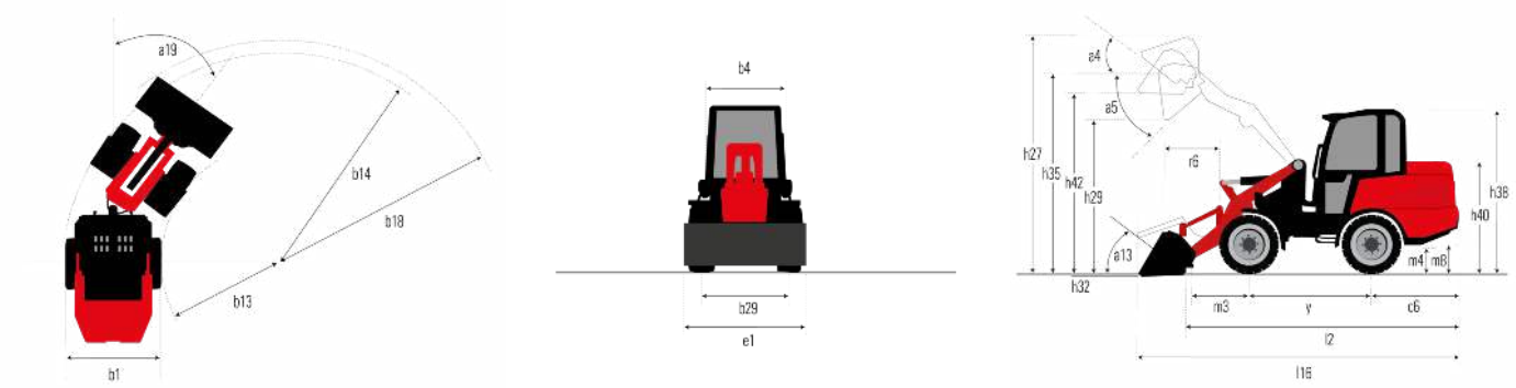
MLA 3-25 H - Tekening met afmetingen
