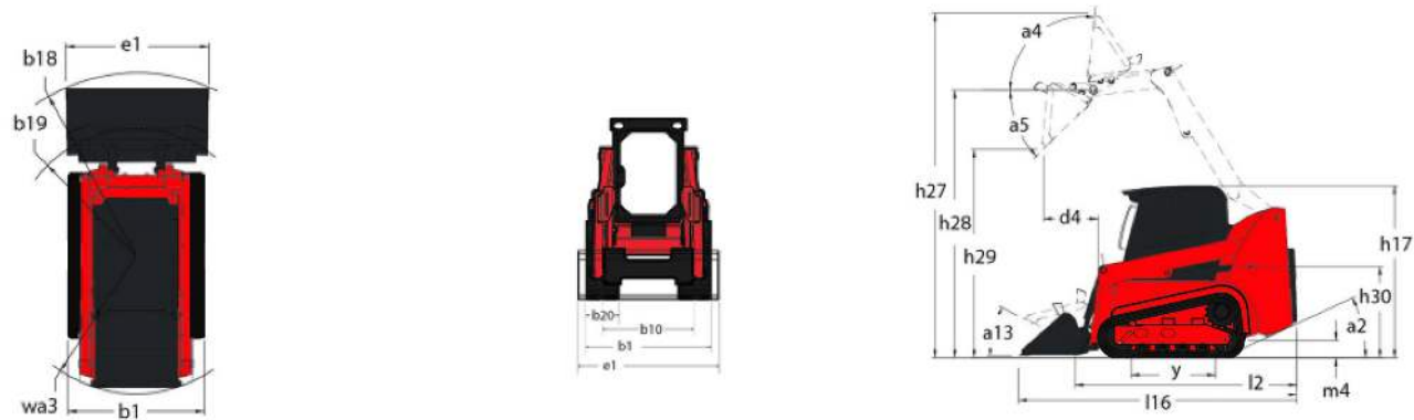
2300VT - Tekening met afmetingen
