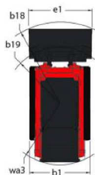
2100VT - Tekening met afmetingen
