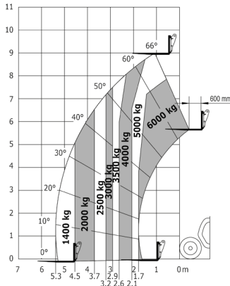
Laaddiagram industrial norm en1459 a Machines op banden met vorken
